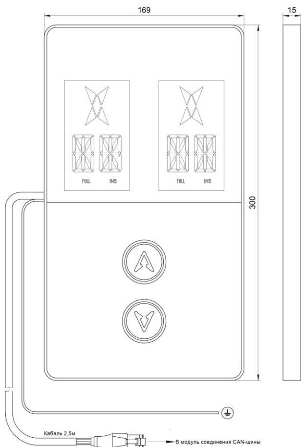
Рис.1 Внешний вид Вызывной пост ОНИКС (жгут RJ45) НШЕК.468381.121
